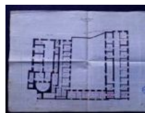
187 Carcere di S. Agata a Bergamo, pianta Secondo piano, s.a., [XIX sec.], Genio Civile XIX secolo, b. 21, fasc. 32, disegno n. 187.
